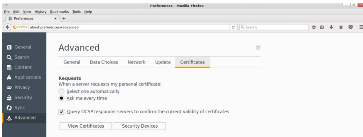
Рис. 45. Вкладка Certificates
