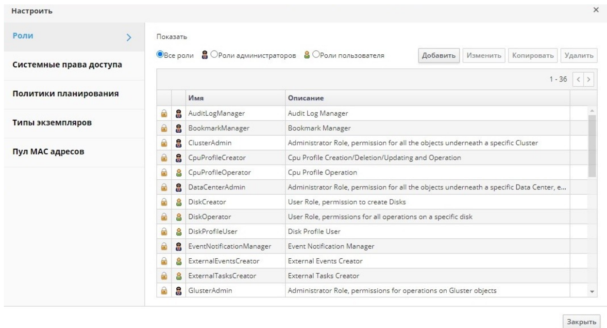
Рис. 1. Настройки системы
