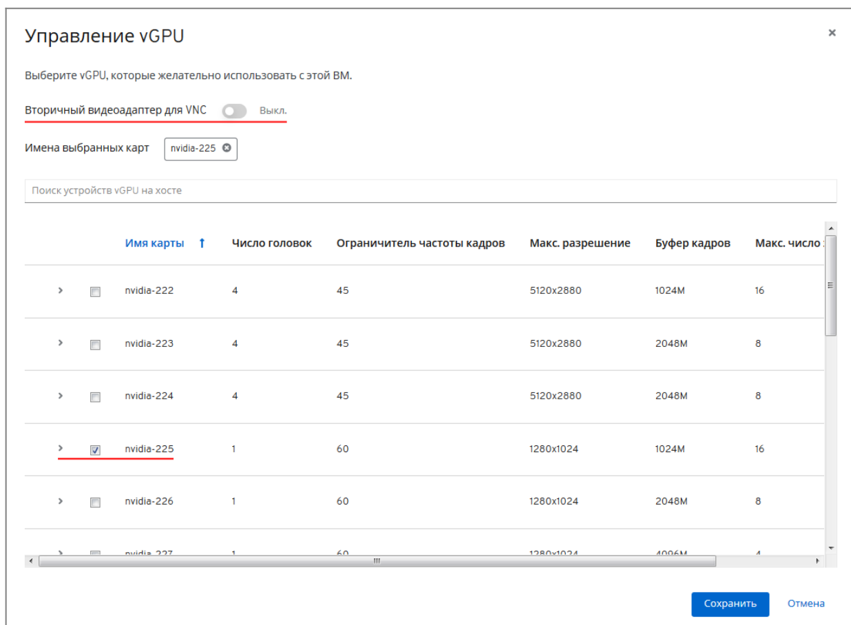
Рис. 52. Управление vGPU
