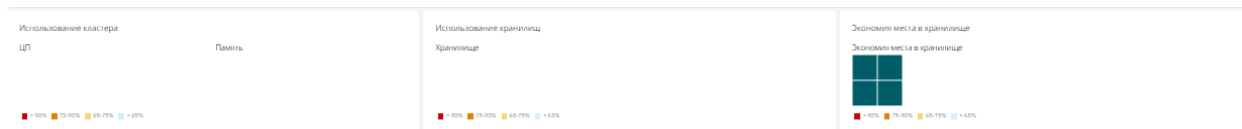
Рис. 16. Общее использование
