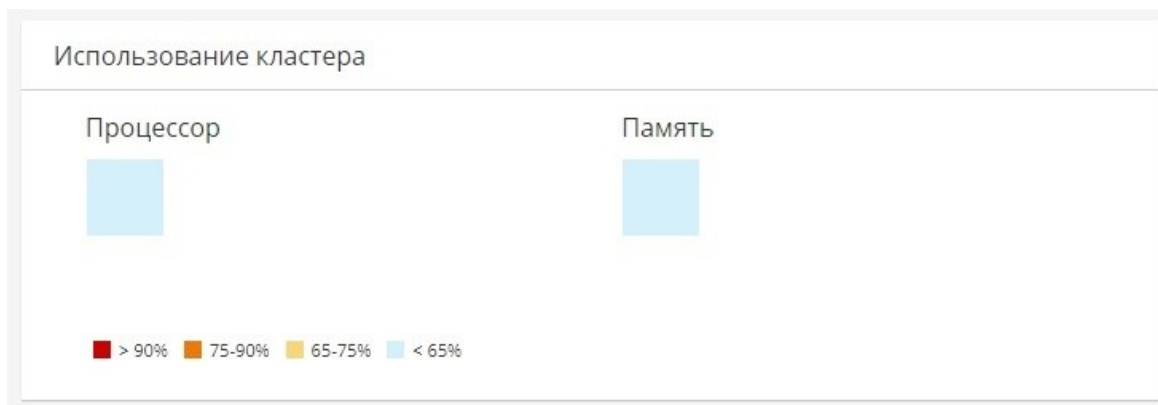
Рис. 18. Использование кластера
