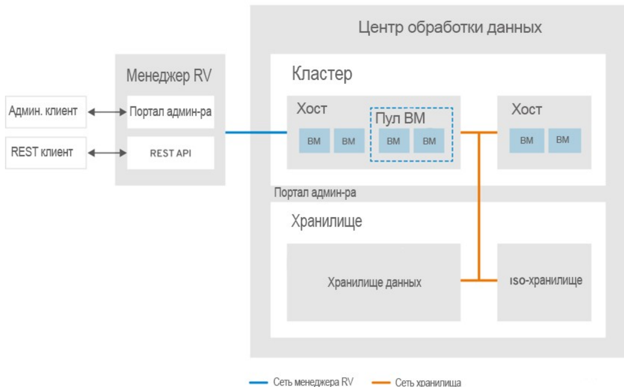
Рис. 30. Кластер
