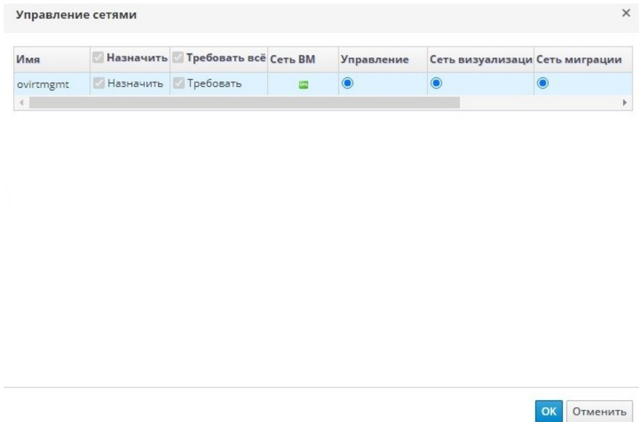
Рис. 34. Управление сетями
