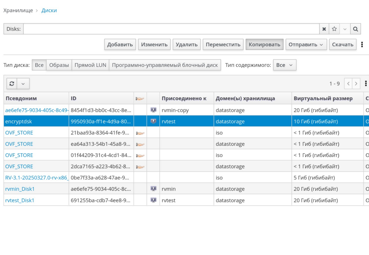
Рис. 163. Общий список дисков в хранилище, с выбранным зашифрованным диском encryptdsk
