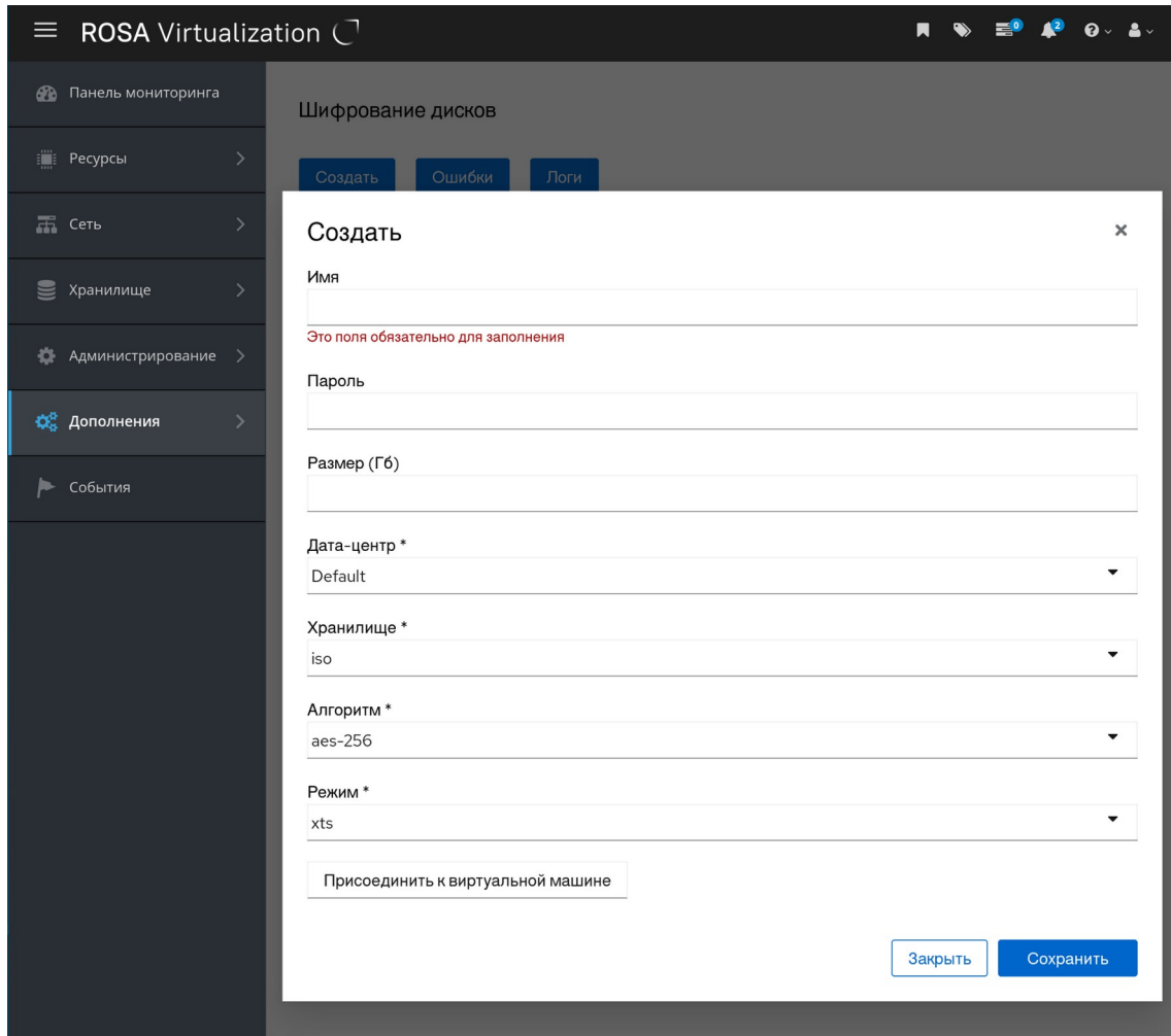
Рис. 156. Создание шифрованного диска
