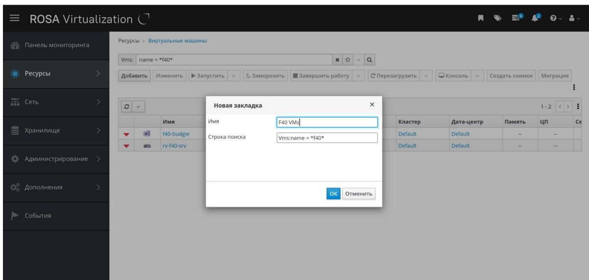
Рис. 54. Форма Новая закладка, для добавления закладки
