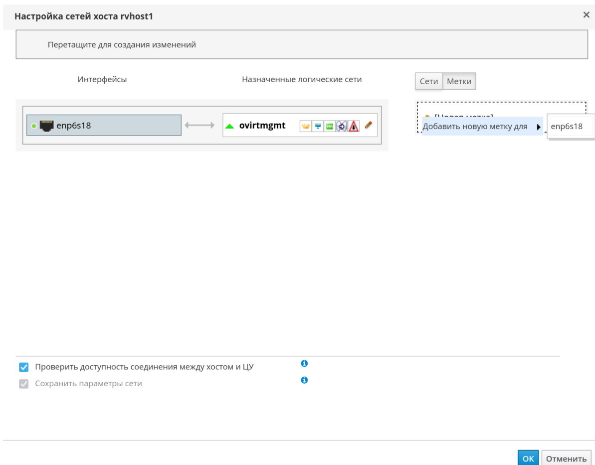
Рис. 123. Выбор интерфейса для добавления новой метки
