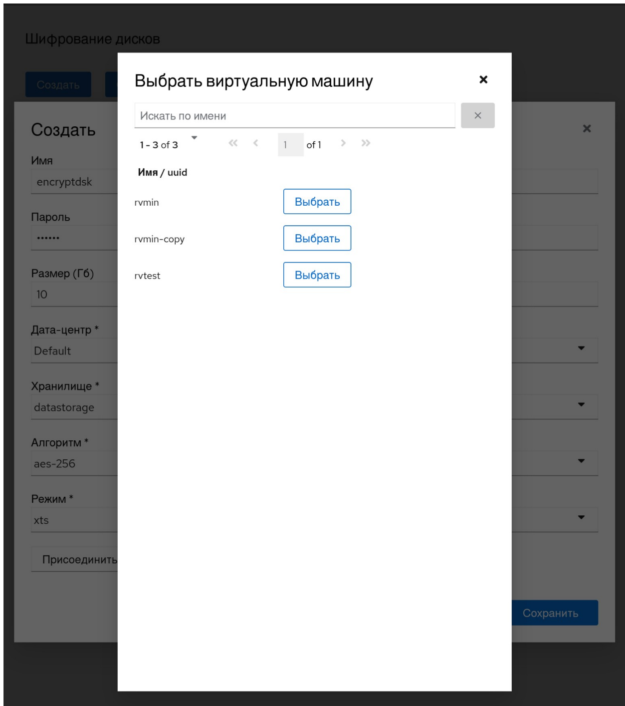
Рис. 161. Выбор ВМ, к которой необходимо присоединить зашифрованный диск
