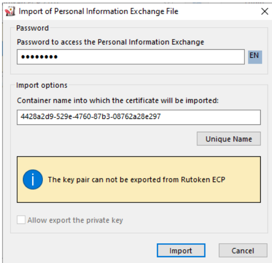
Рис. 180. Ввод пароля для файла
