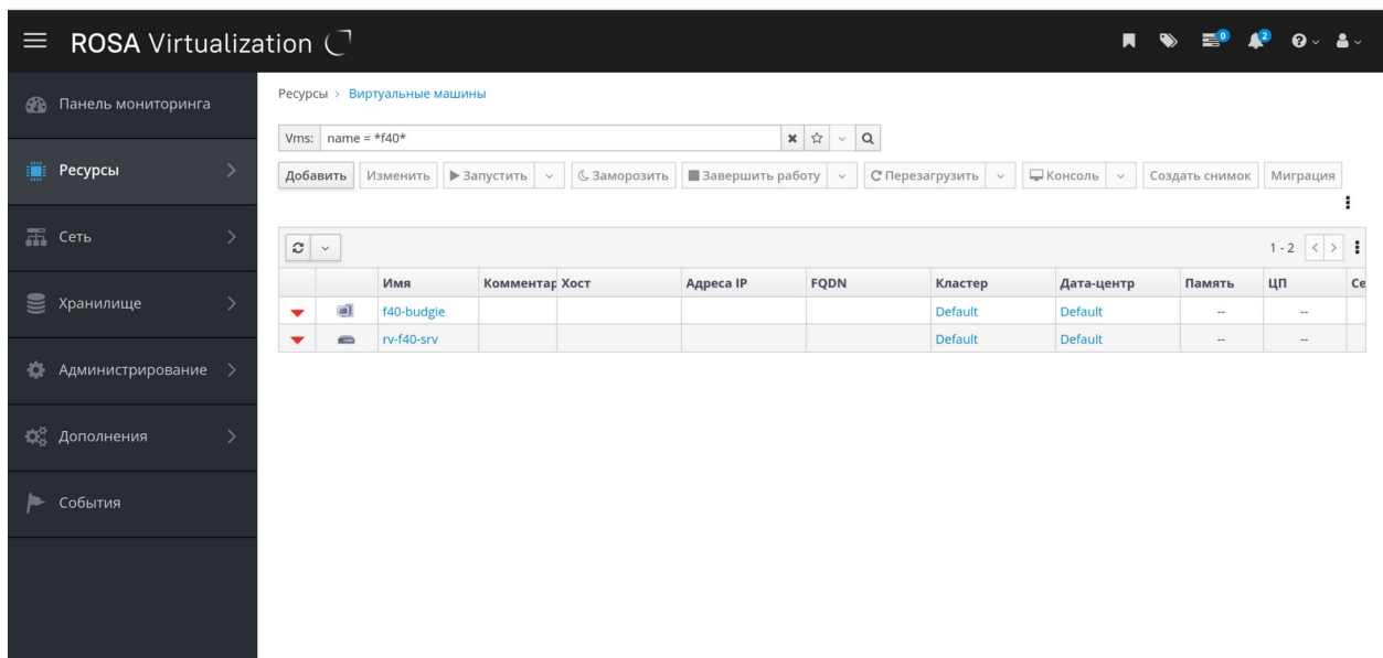
Рис. 50. Поиск VM по шаблону имени
