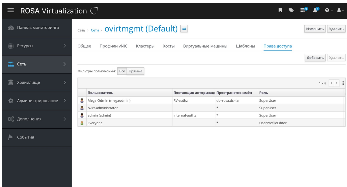
Рис. 119. Вкладка Права доступа
