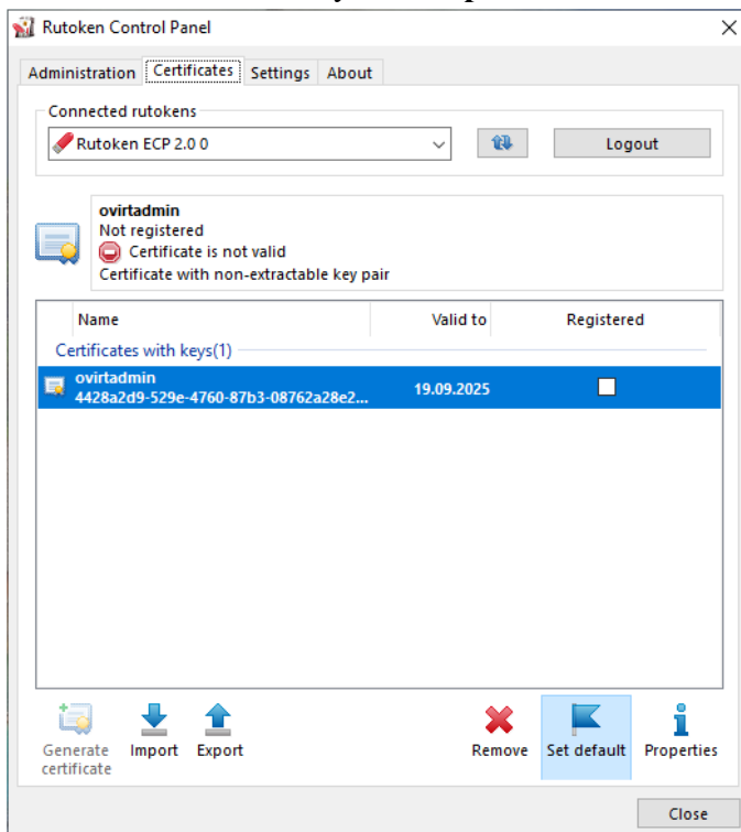
Рис. 179. Контрольная панель Рутокен – вкладка Сертификаты
