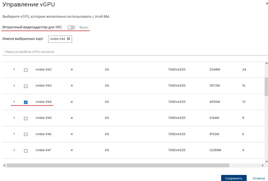
Рис. 187. Настройка vGPU
