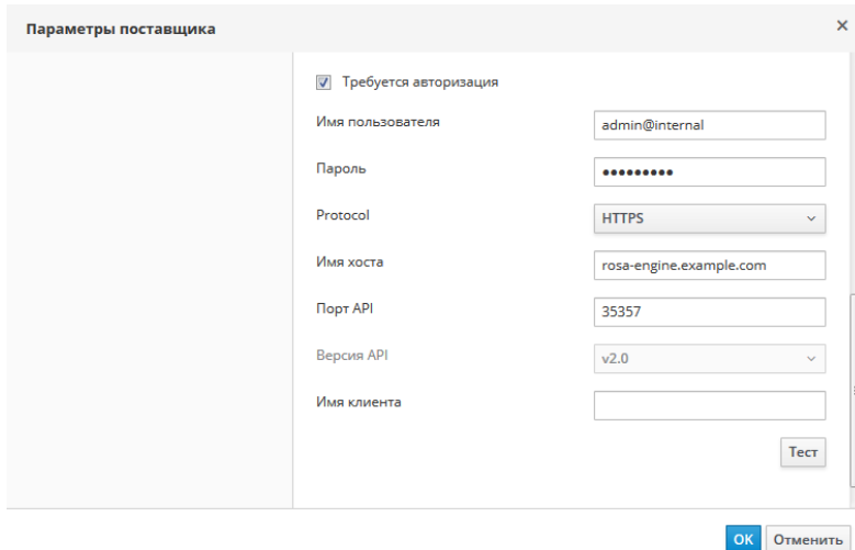
Рис. 178. Окно «Параметры поставщика»
