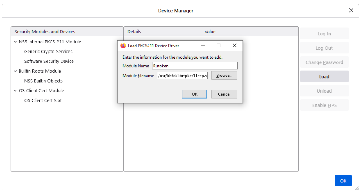
Рис. 183. Настройки браузера с библиотеками библиотекой PKCS#11
